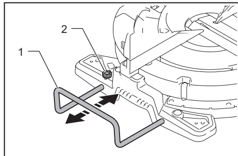
► 1. Holder 2. Screw
