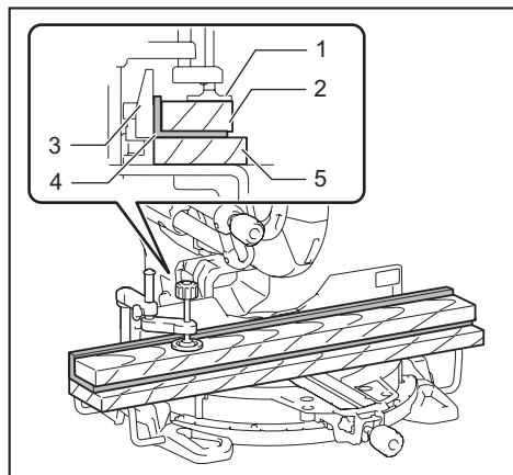
► 1. Étau 2. Cale d'espacement 3. Garde de guidage 4. Profilé d'aluminium 5. Cale d'espacement
